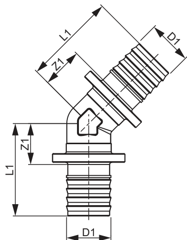
TECEflex 45° elbow
